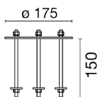
Placa de cajón de acero galvanizado pintado - Apto para base de suelo
