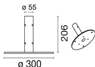
Base para mástil de suelo de 60 mm- Adecuada para mástil H-3m
