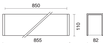
VERSIONE CON 2 STRISCE LED VERSION WITH 2 STRIPS
