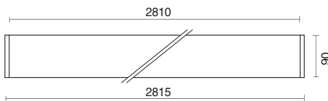
L. 2810 mm = solo apparecchio - only fixture L. 2815 mm = apparecchio + testate - fixture + caps
