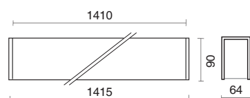
L. 1410 mm = solo apparecchio - only fixture L. 1415 mm = apparecchio + testate - fixture + caps
