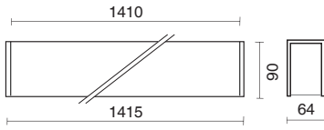
L. 1410 mm = solo apparecchio - only fixture L. 1415 mm = apparecchio + testate - fixture + caps
