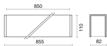
L. 850 mm = solo apparecchio - only fixture L. 855 mm = apparecchio + testate - fixture + caps
