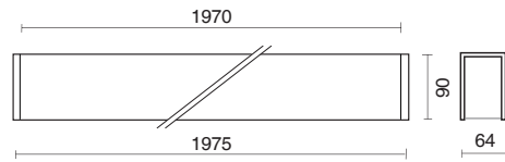
L. 1970 mm = solo apparecchio - only fixture L. 1975 mm = apparecchio + testate - fixture + caps
